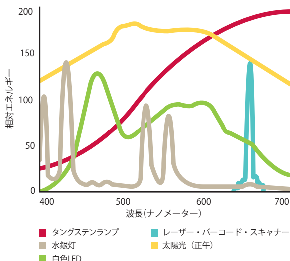
一般的な可視光源のスペクトル
